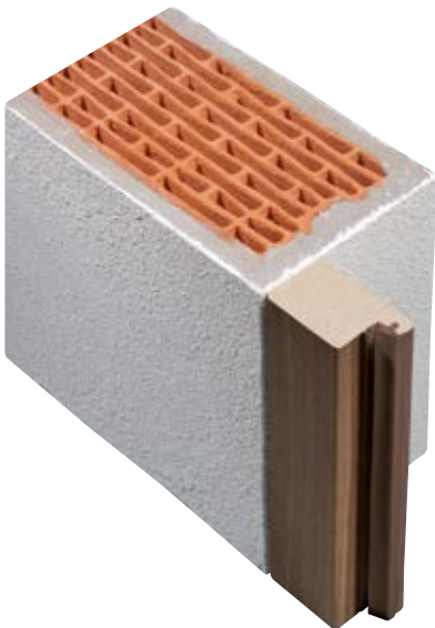
BLENDRAHMEN BM 43/65 in der Laibung montiert (beliebige Position)
