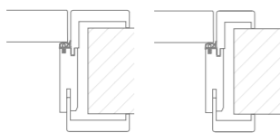
S-DESIGN-FB Türblatt stumpf, öffnet nach außen:
